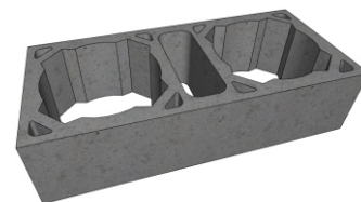
TVÁRNICE P2+š 360x810x200 mm
