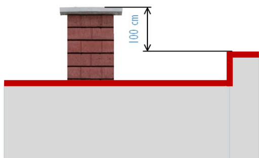
Obr. 4 Vyústění komínu nad plochou střechou
