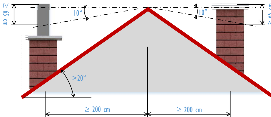
Obr. 2 Způsob vyústění komínů nad šikmou střechou vzdálenost vyústění od hřebene nad 200 cm
