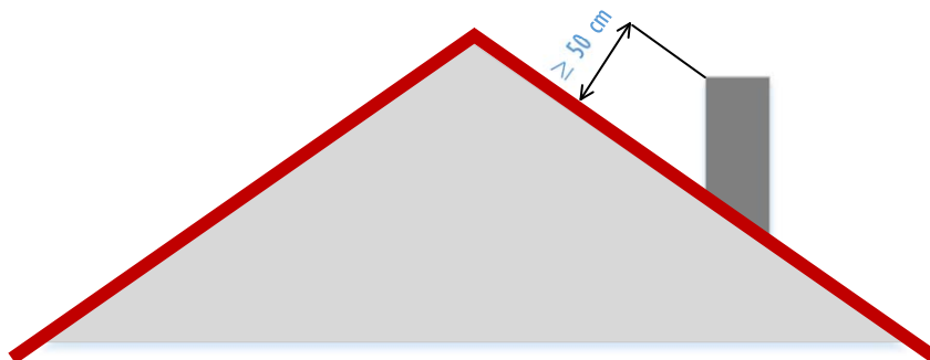
Obr. 3 Vyústění přetlakového komínu a komínu s umělým tahem nad šikmou střechou
