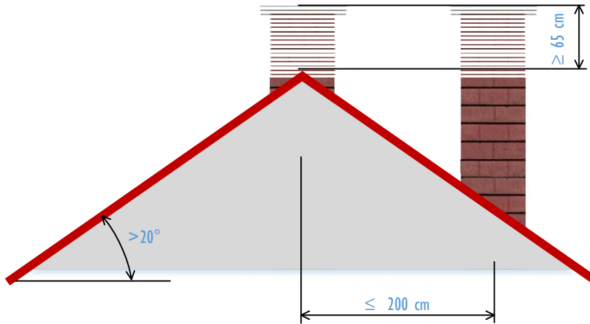
Obr. 1 Způsob vyústění komínů nad šikmou střechou vzdálenost vyústění od hřebene do 200 cm
