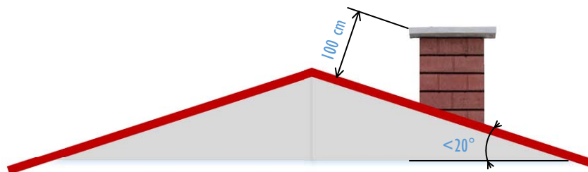
Obr. 5 Vyústění komínu nad plochou střechou (sklone menší než 20°)
